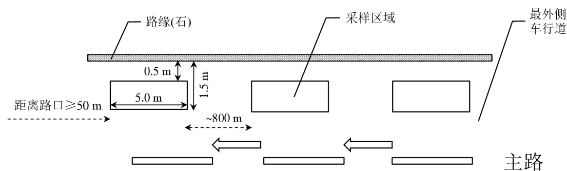
图1 道路扬尘采样示意图
